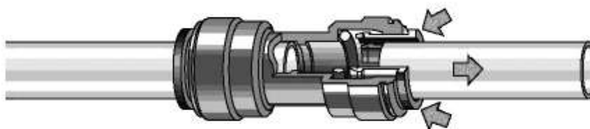
Entfernen von Schläuchen aus Quick-Verbinder (Ring hineindrücken und Schlauch herausziehen)
